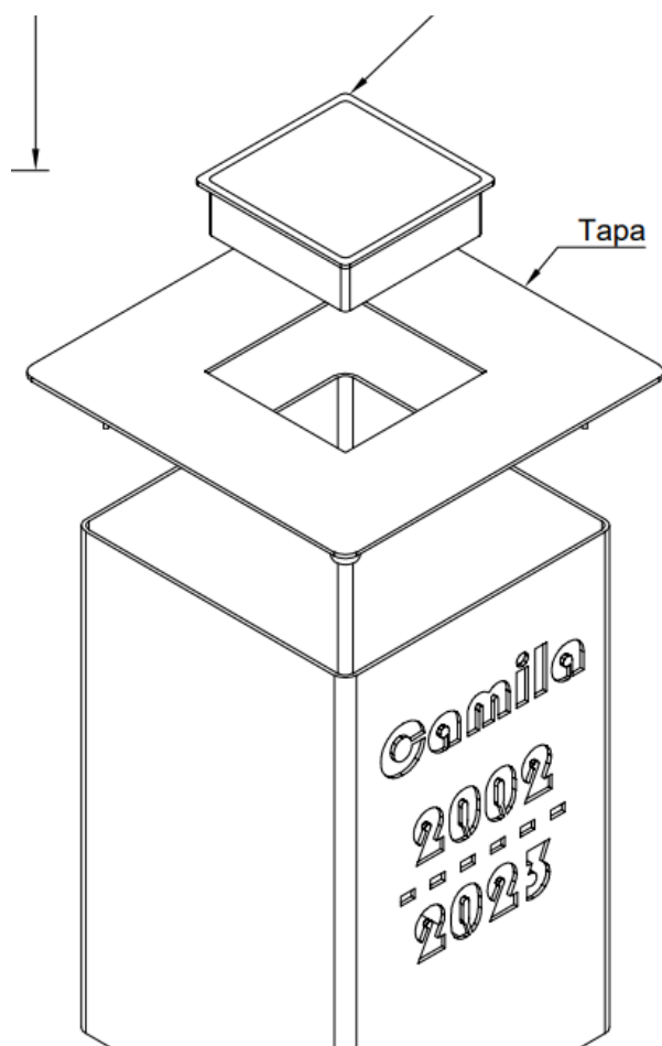
Detalle de los componentes para aprobación del cliente
